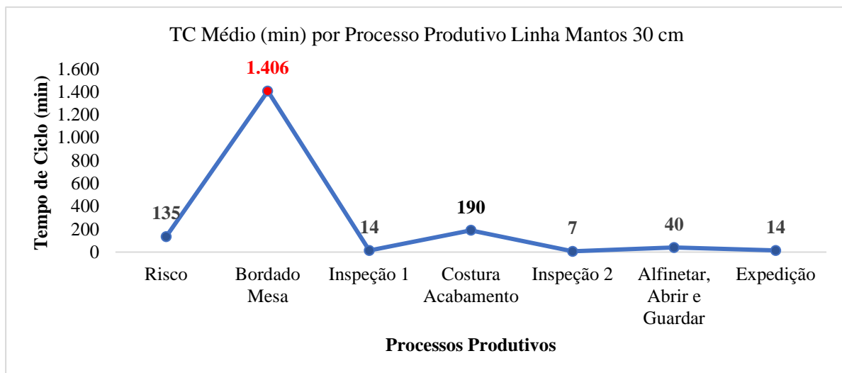
Gráfico 1 – Tempo de Ciclo Médio (min) por Processo Produtivo Linha Mantos 30 cm. Fonte: Elaborado pelo próprio autor.
